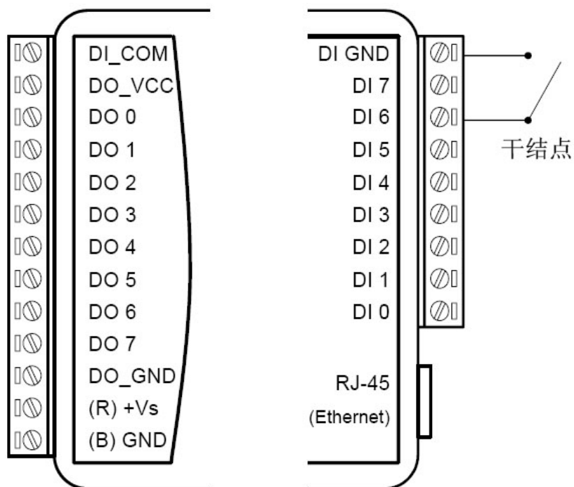
图 1.2 RemoDAQ-8352 干结点数字输入
