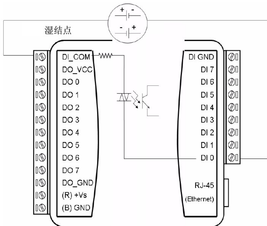
图 1.3 RemoDAQ-8352 湿结点数字输入
