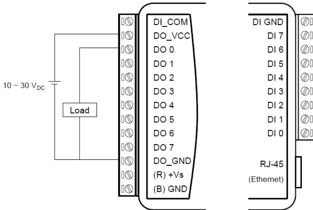
图 1.4 RemoDAQ-8352 源点型数字输出
